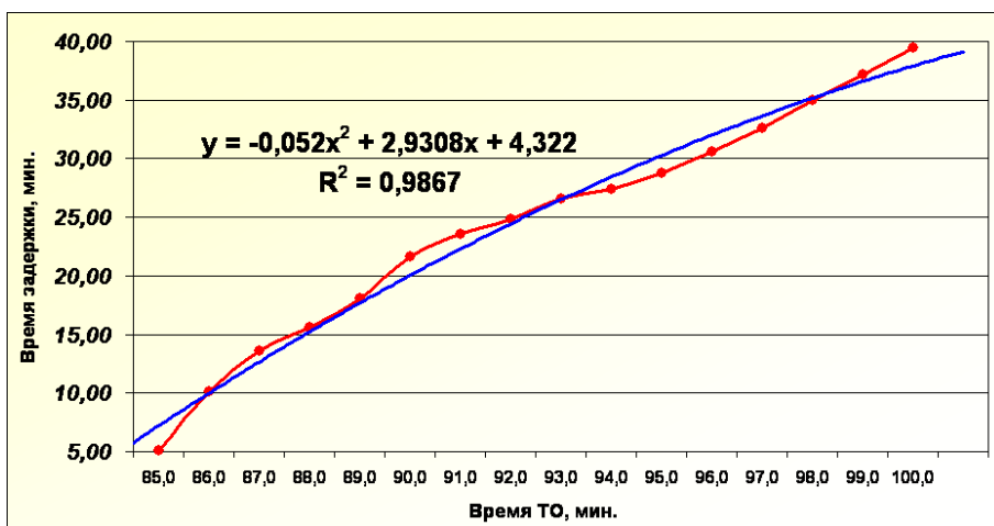
Рис. П1.2. Зависимость времени задержки рейса от времени технического обслуживания ВС
